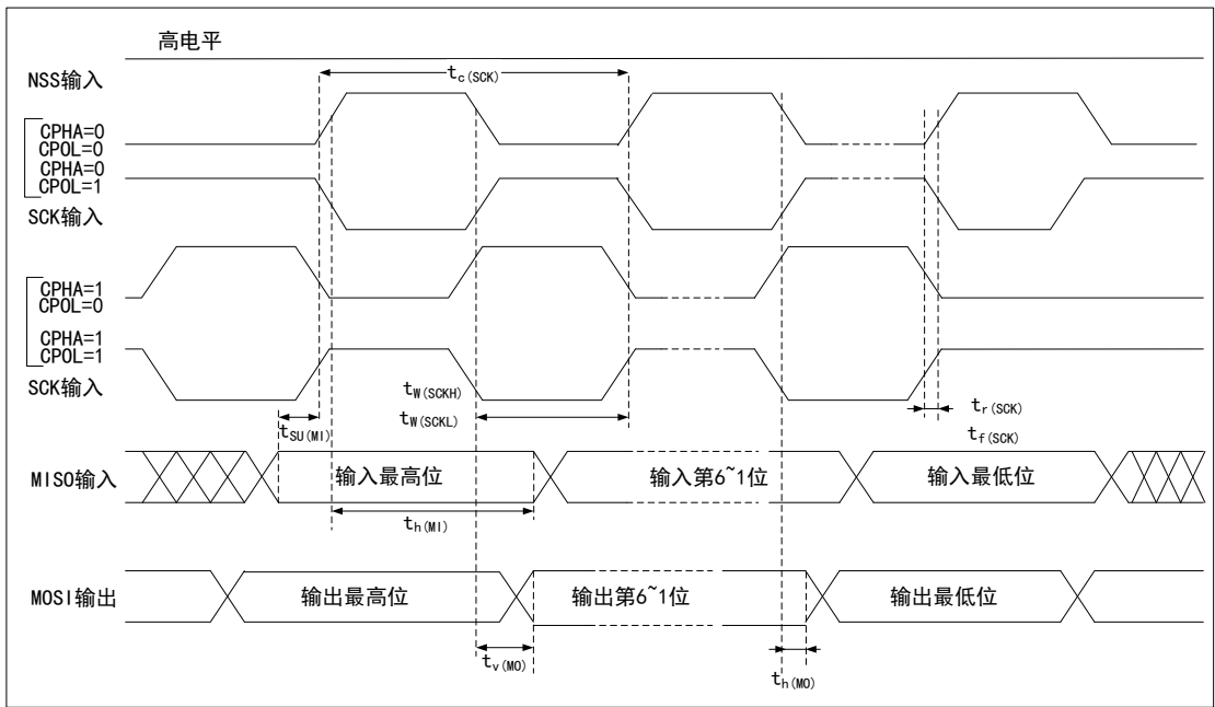
图11 SPI 时序图—主模式
